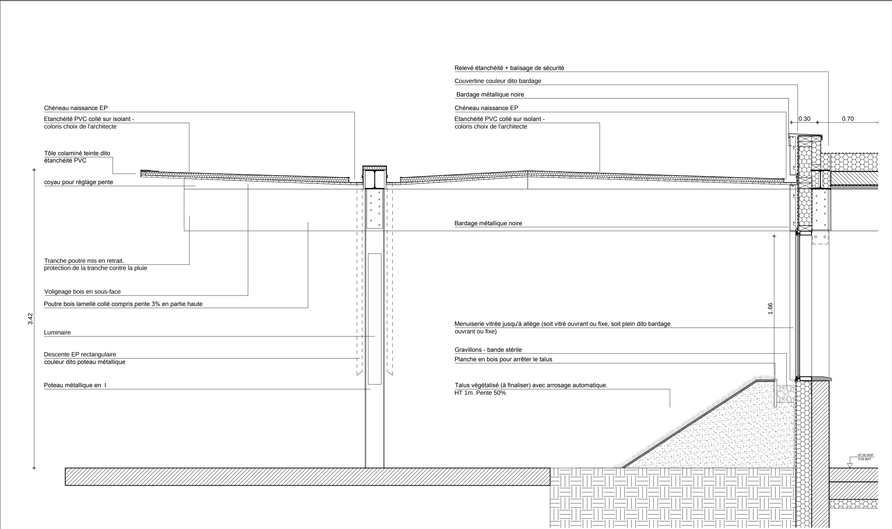
Coupe sur préau élémentaire 1/25
