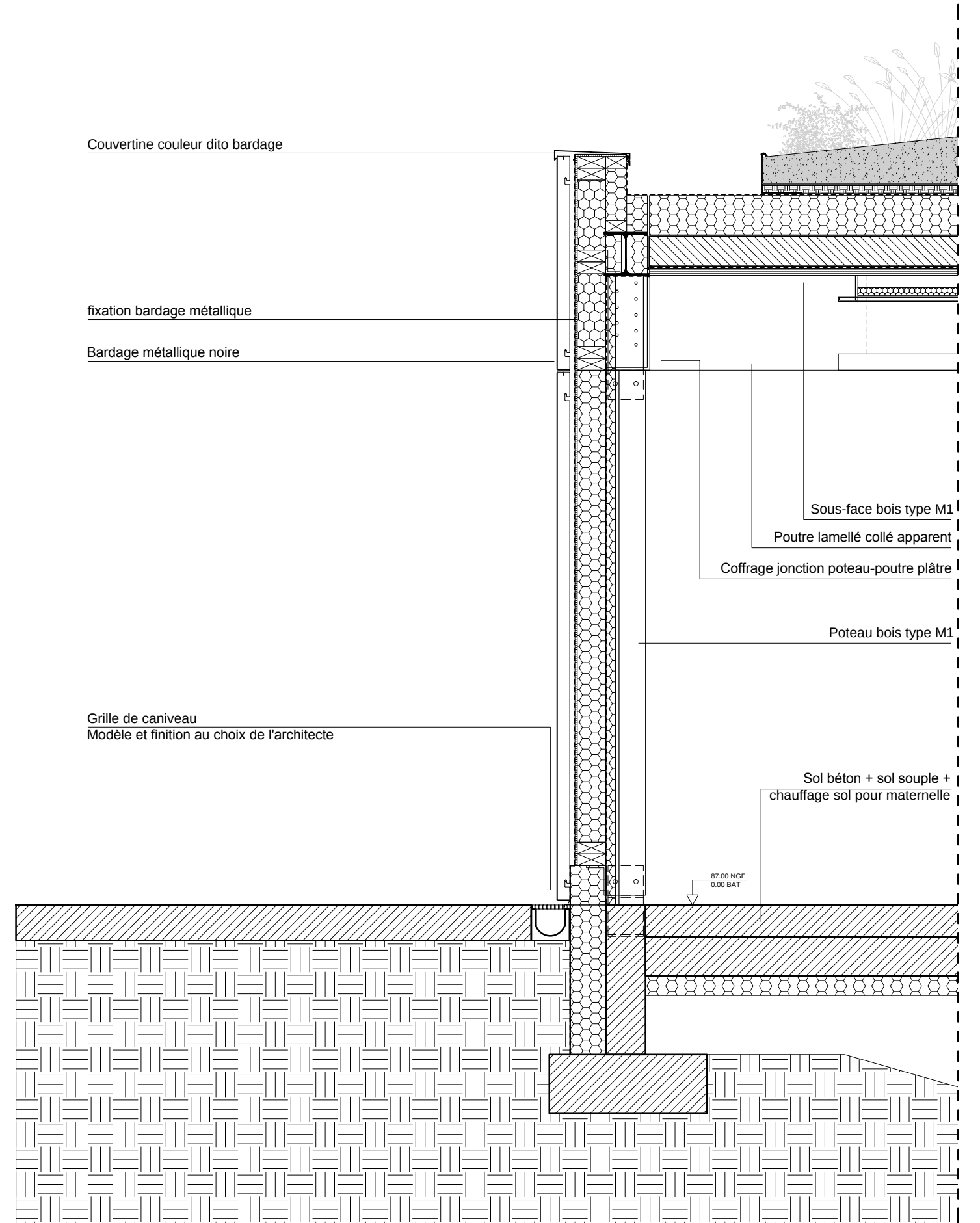
Composition façade ossature bois Bardage toute hauteur 1/25
