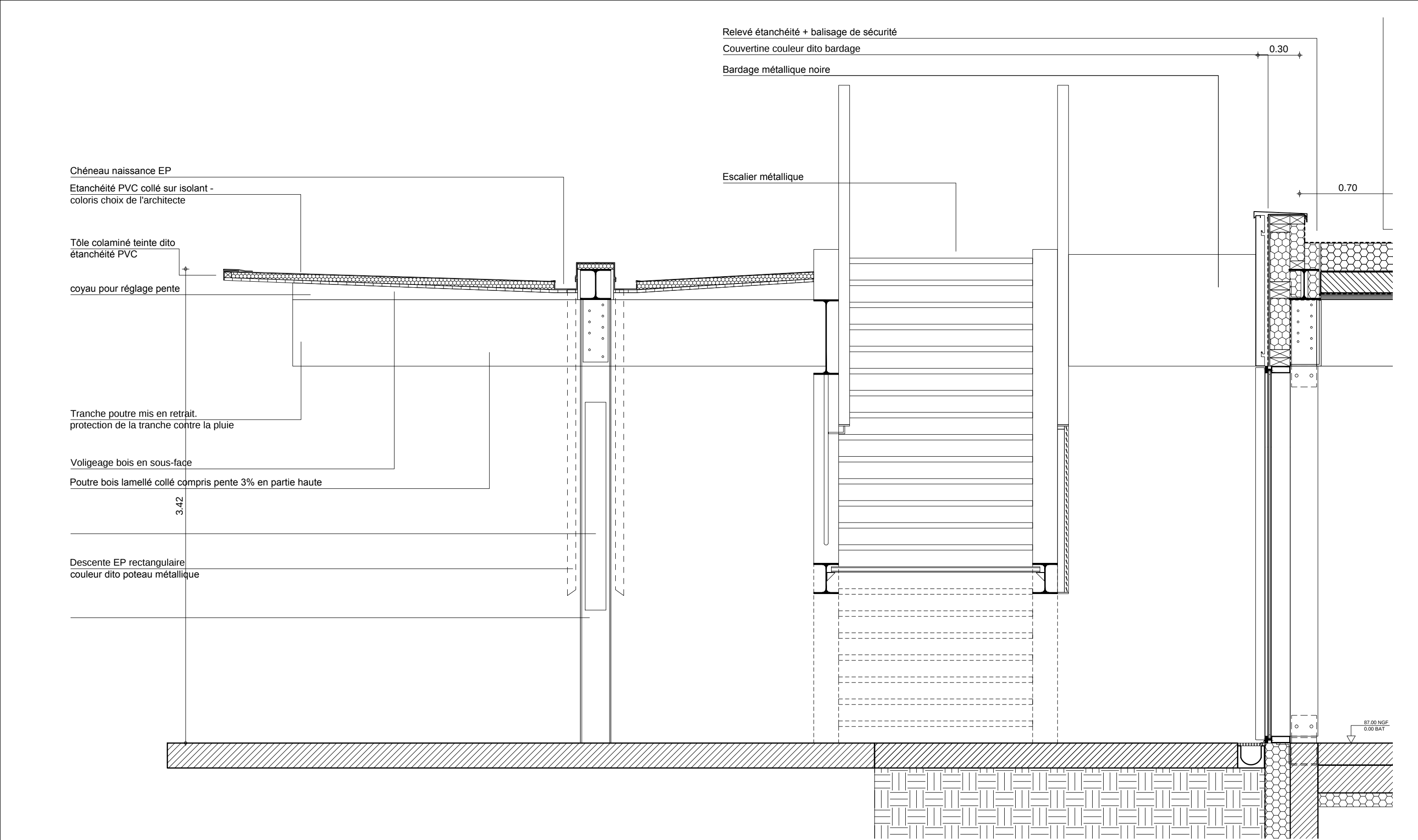
Coupe sur préau élémentaire Escalier 1/25
