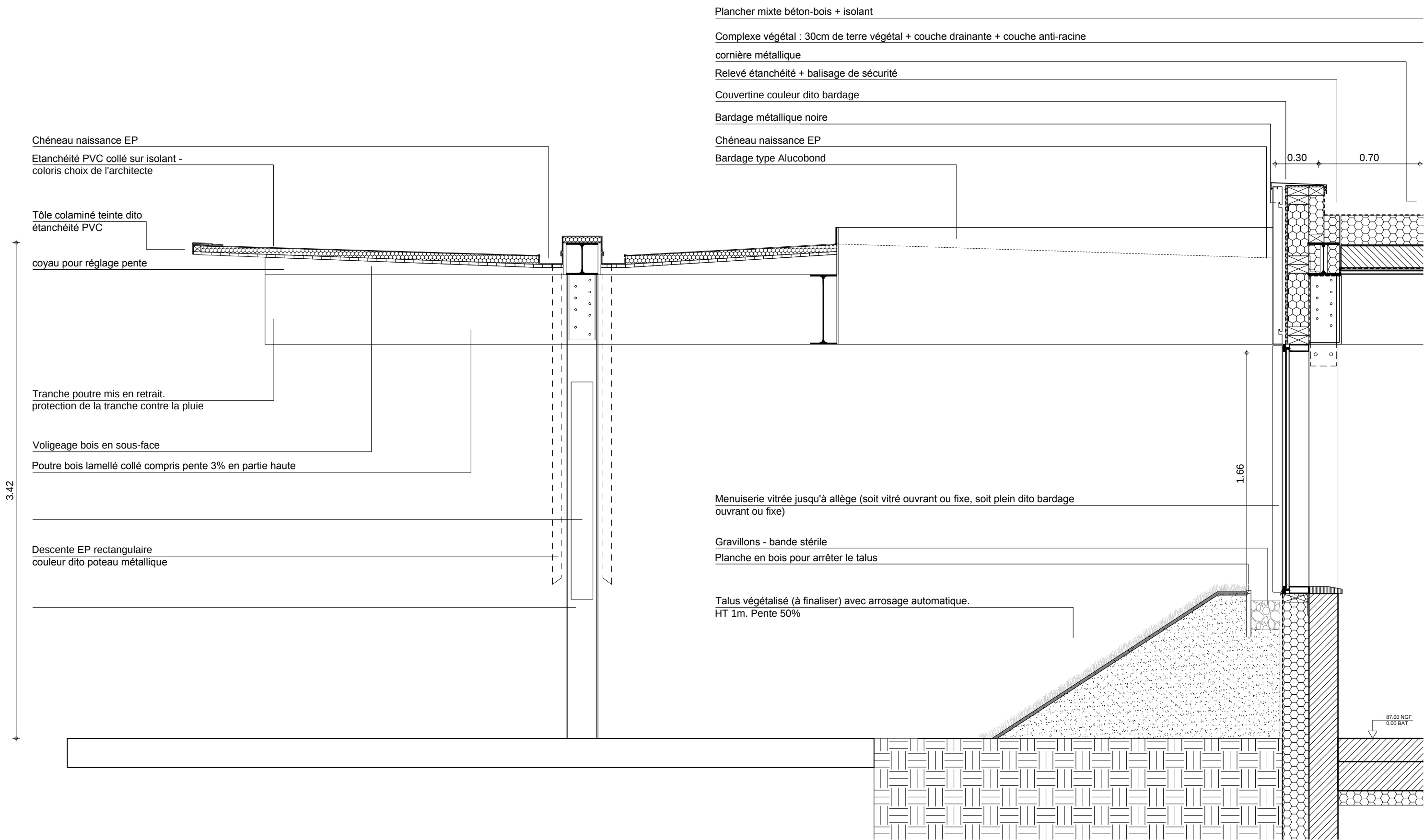
Coupe sur préau élémentaire Puits de jour 1/25
