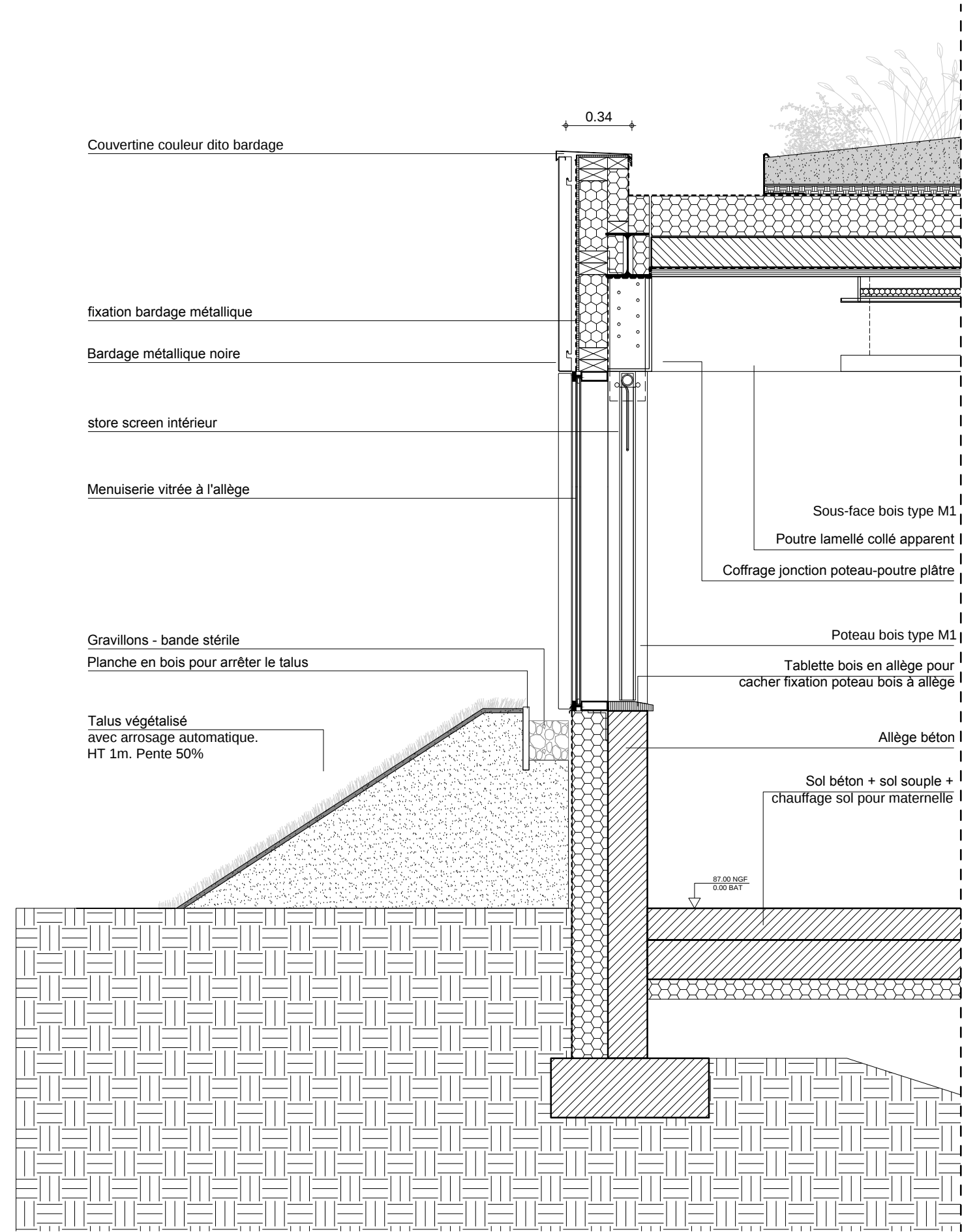
Composition façade ossature bois Vitrage + store intérieur sur allège 1/25
