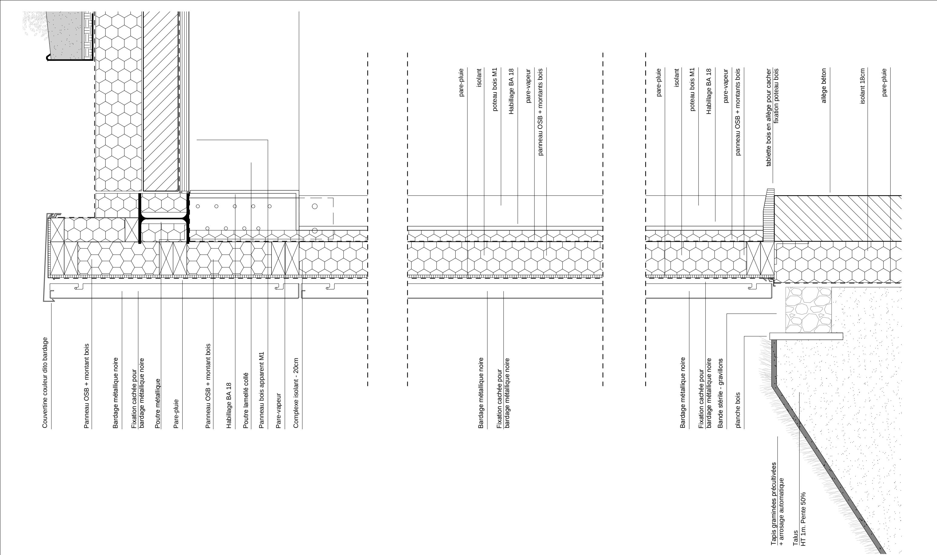
Composition façade ossature bois Bardage plein sur allège 1/25
