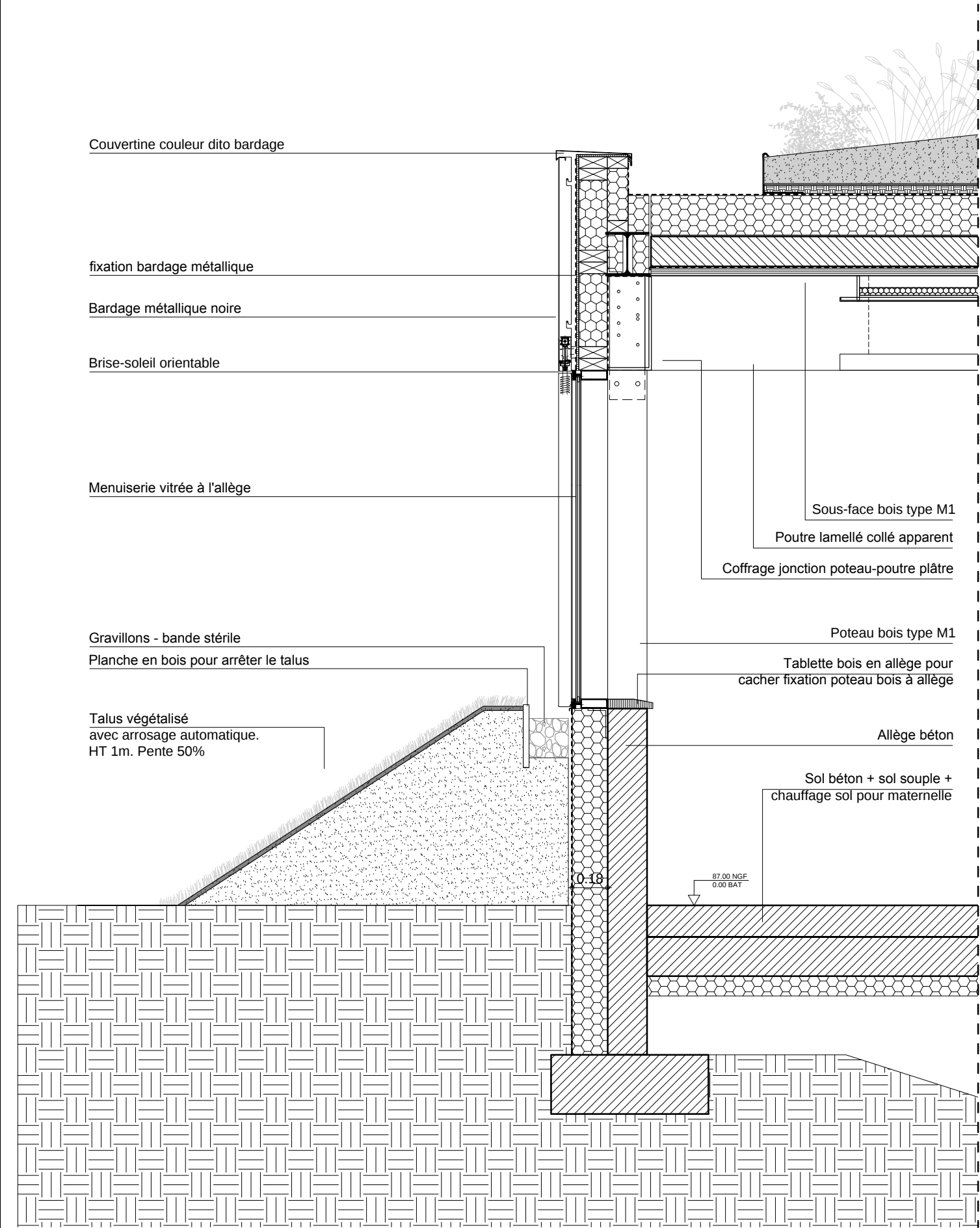
Composition façade ossature bois Vitrage + BSO sur allège 1/25
