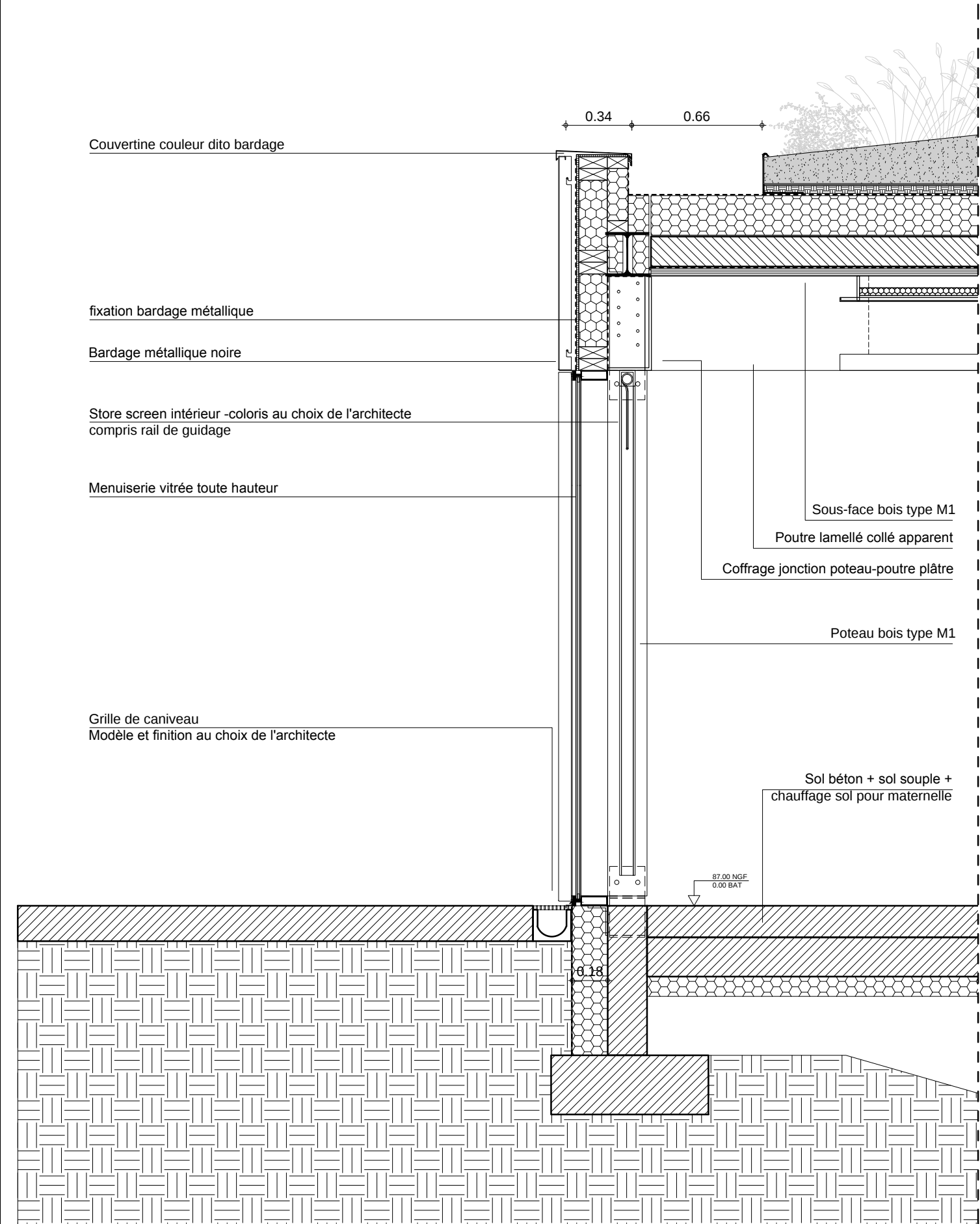
Composition façade ossature bois Vitrage toute hauteur 1/25
