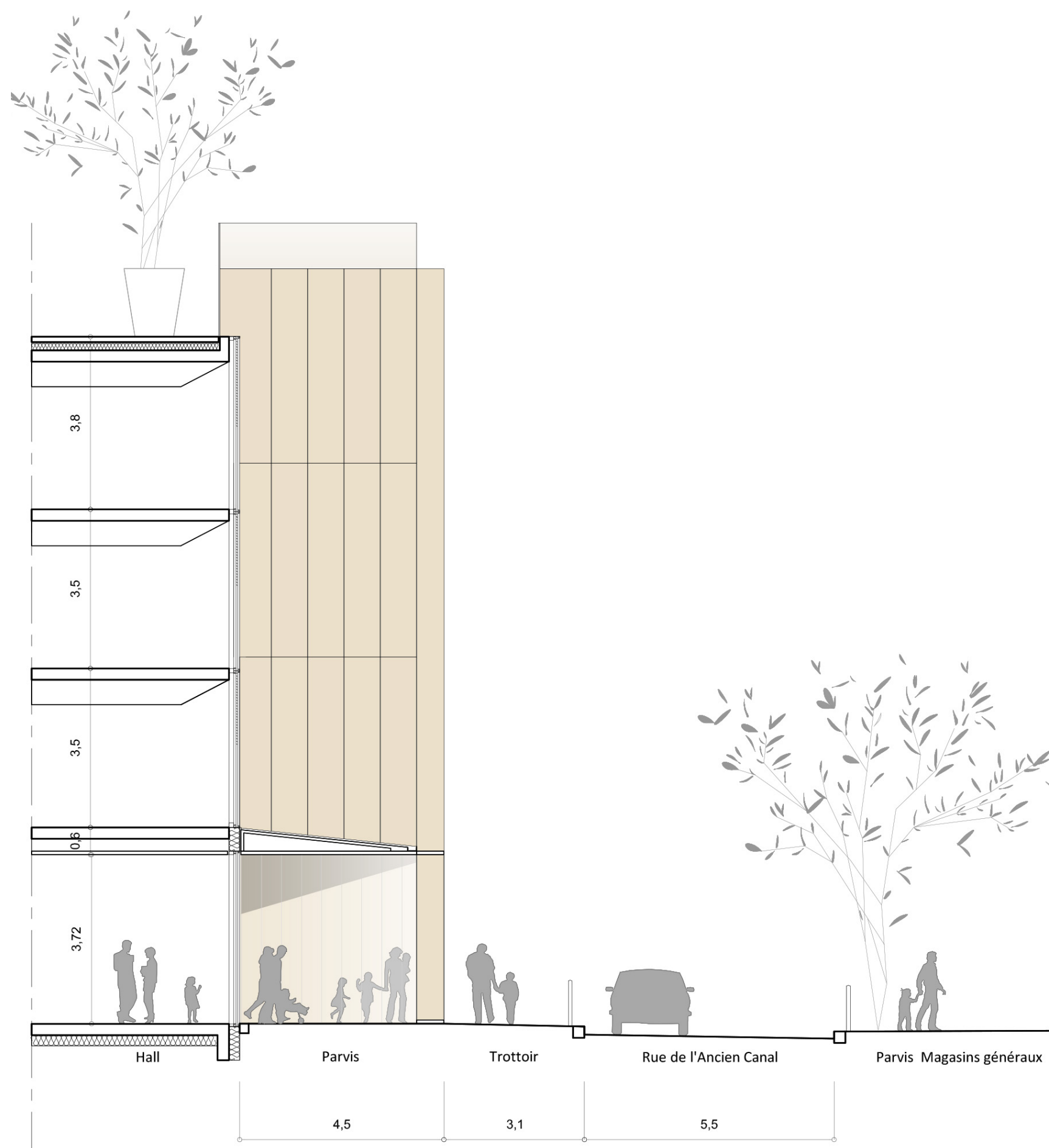
COUPE ET FACADE SUR L'ENTREE
